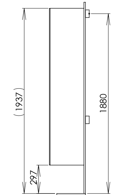
Högskåp/High cabinet/Korkeakaappi
