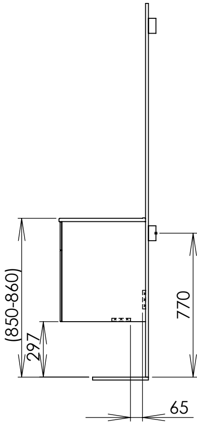
Underskåp/Vanity unit/Allaskaapit
