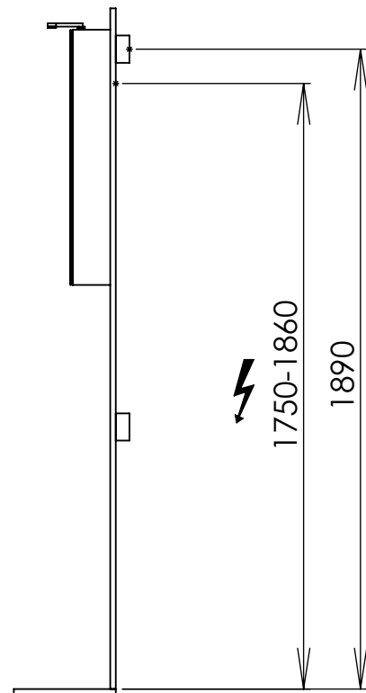
Spegelskåp/Mirror cabinet/Peilikaapit
